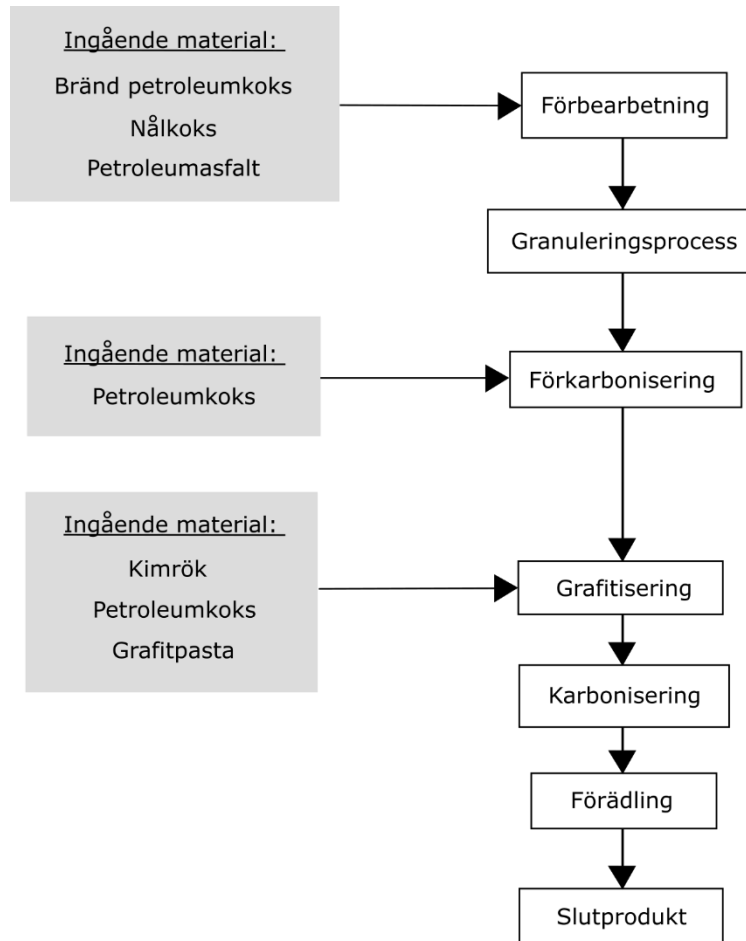
Figur 5. Produktionsprocess av anodmaterial.
